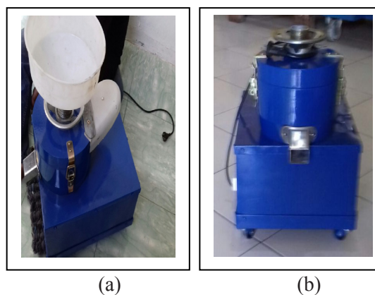
Gambar 3 (a) dan (b) mesin pemeras/penghalus bahan baku jamu yang telah 100% jadi, yang (a) dengan menggunakan cerobong untuk memasukkan bahan baku jamu
