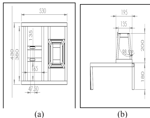
Gambar 2. (a) dan (b) Desain dan ukuran mesin pemeras/penghalus bahan baku jamu beserta dudukannya
